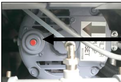
Commutateur de réarmement de la pompe du filtre
